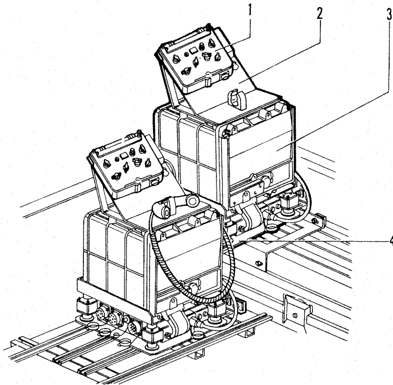
Bild 77 Einbau des 2. Funkgerätes (hier SEM 25)
